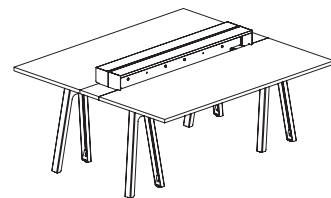
SINGOLA CONTRAPPPOSTA SINGLE MODULE INDIVIDUEL FACE A FACE L. 180/200 - P. 160
